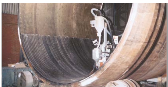
Separator Vessel (Nickel alloy 400) Soudotape NiCu7 + Record EST 400
